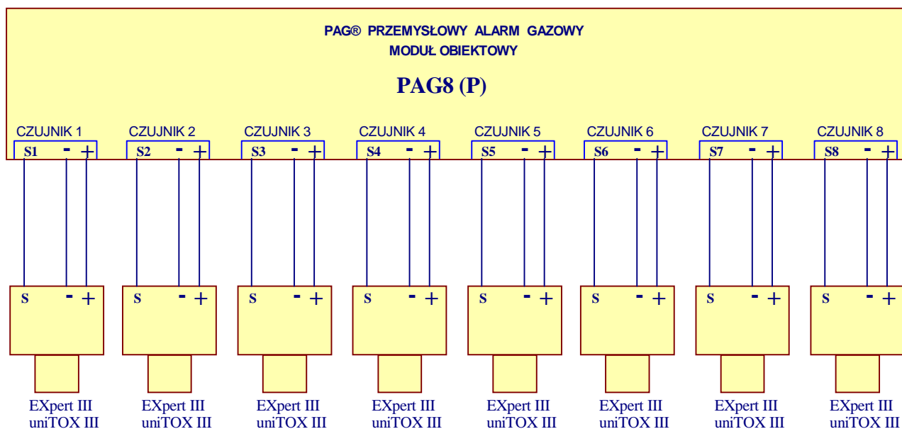
Rys.4. Podłączenie Uniwersalnej Głowicy Gazometrycznej „EXpert III” do Modułu Obiektowego PAG8 (P).
