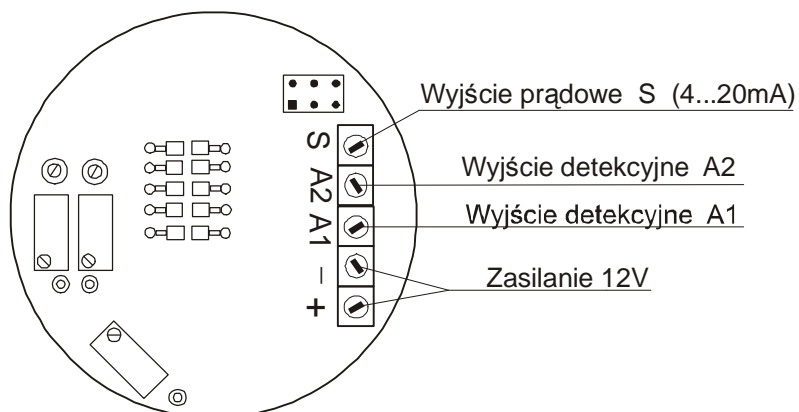
Rys.2. Listwa zaciskowa Uniwersalnej Głowicy Gazometrycznej „EXpert III”
