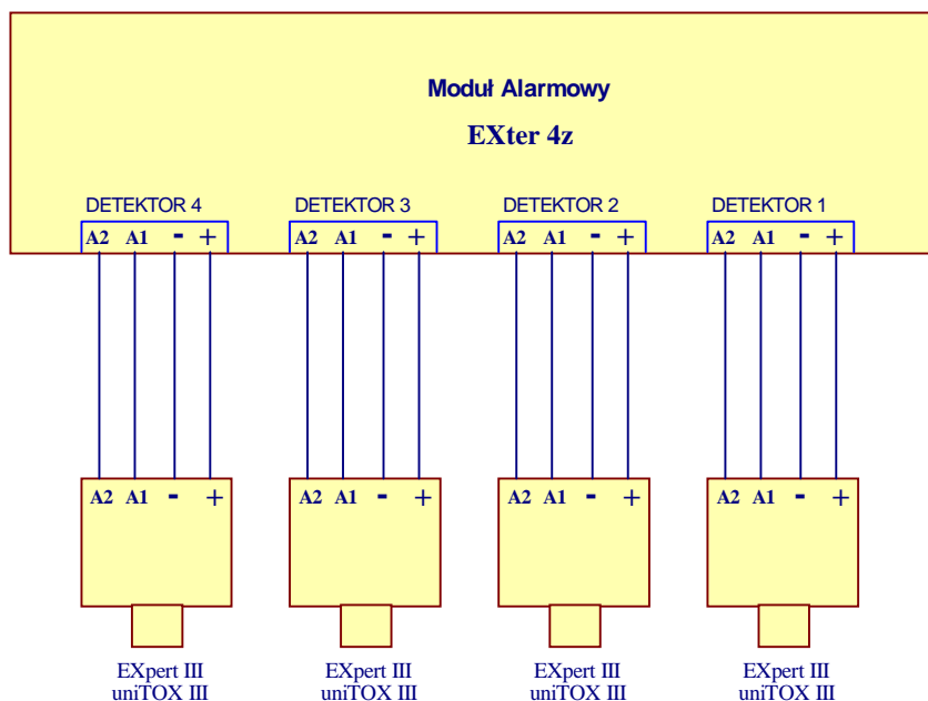
Rys.3. Podłączenie Uniwersalnej Głowicy Gazometrycznej „EXpert III” do Modułu Alarmowego Exter 4z
